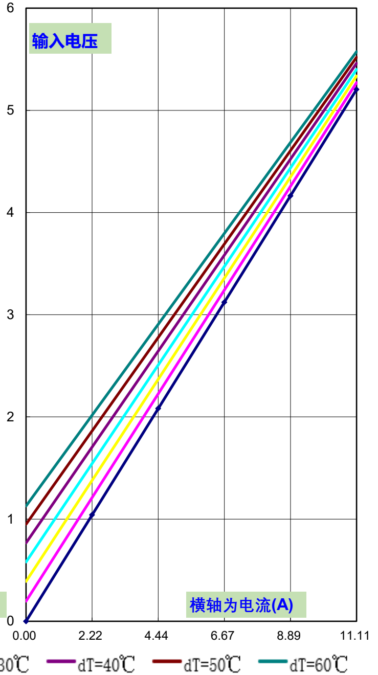
电压/电流曲线
